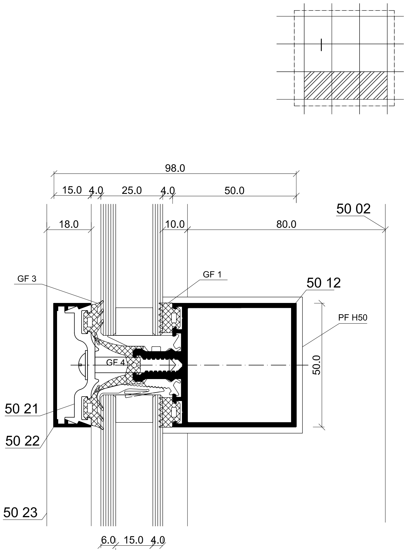
Vertikalni presek KONTINUALNE fasade
