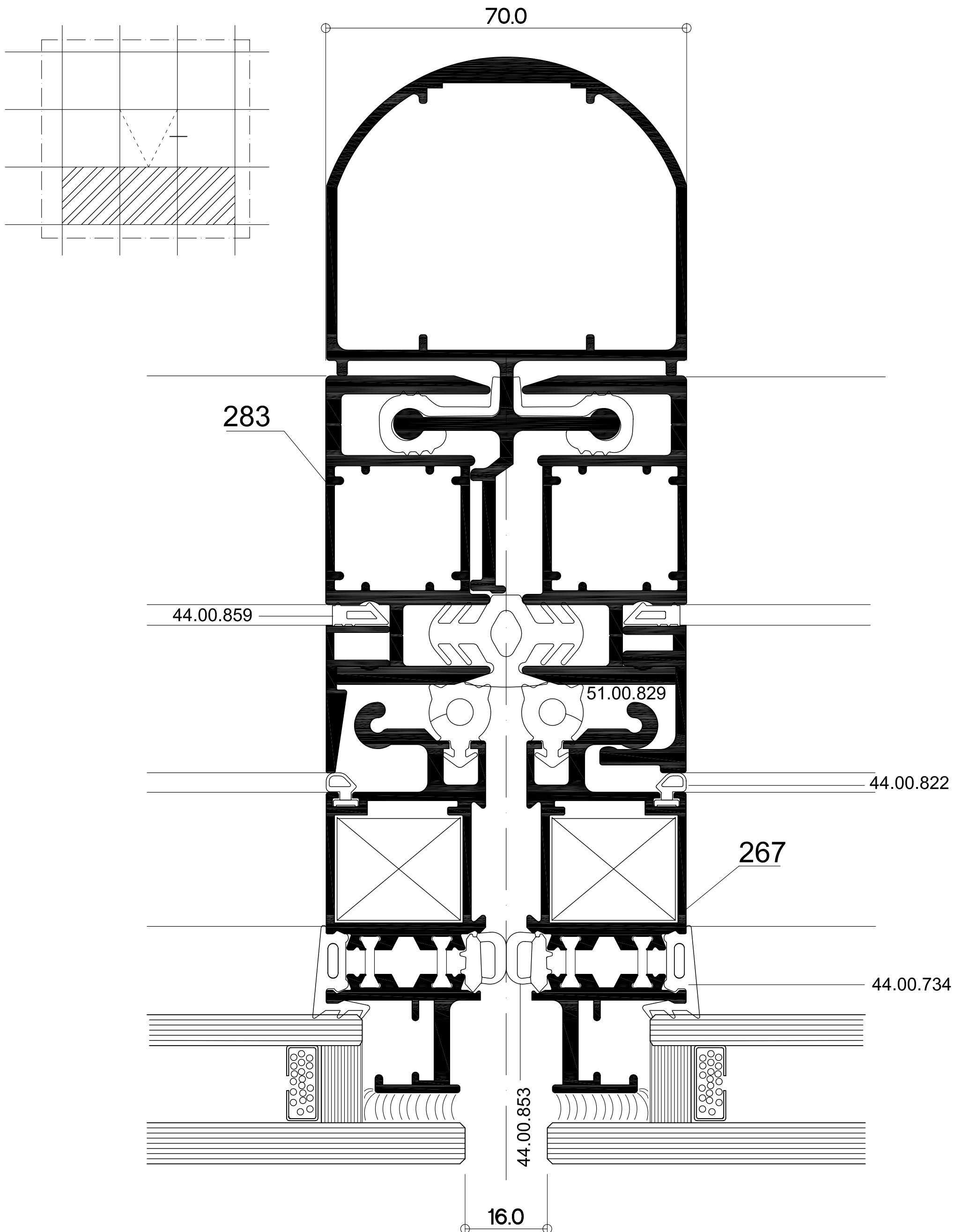
Horizontalni presek STRUKTURALNE fasade
